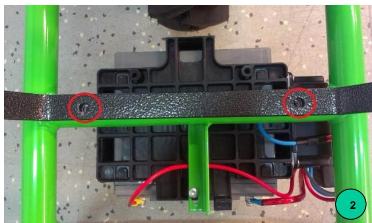
Obr.2: Odšroubujeme korbu/nástavbu z rámu Motúčka a přiložíme nástavbu pro včelaře. Za použití stejných šroubů nástavbu upevníme
